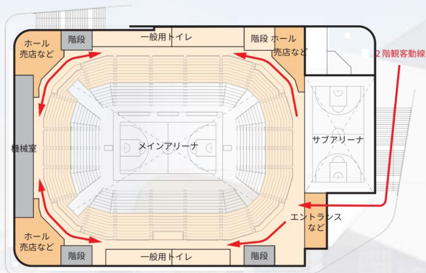
2階平面イメージ (案)
